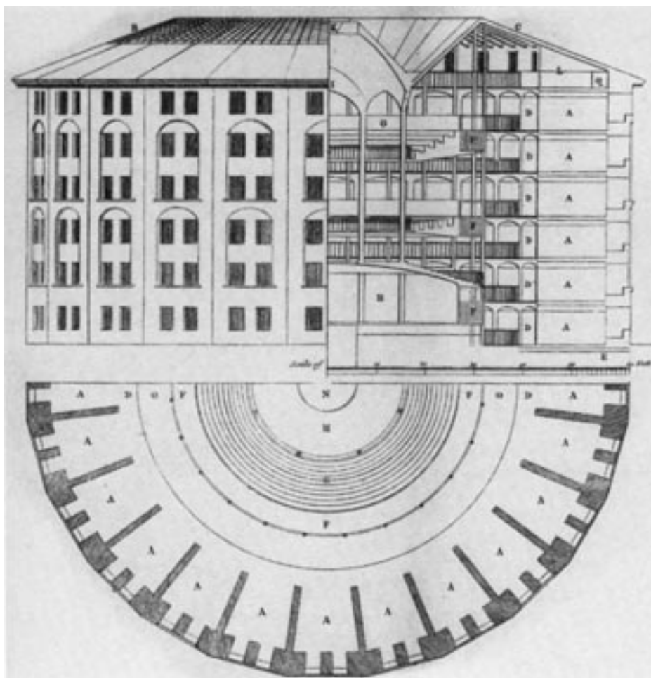
Nákres věznice postavené podle panoptického systému, Jeremy Bentham, 1791.
