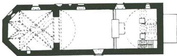
Pôdorys podlažia
